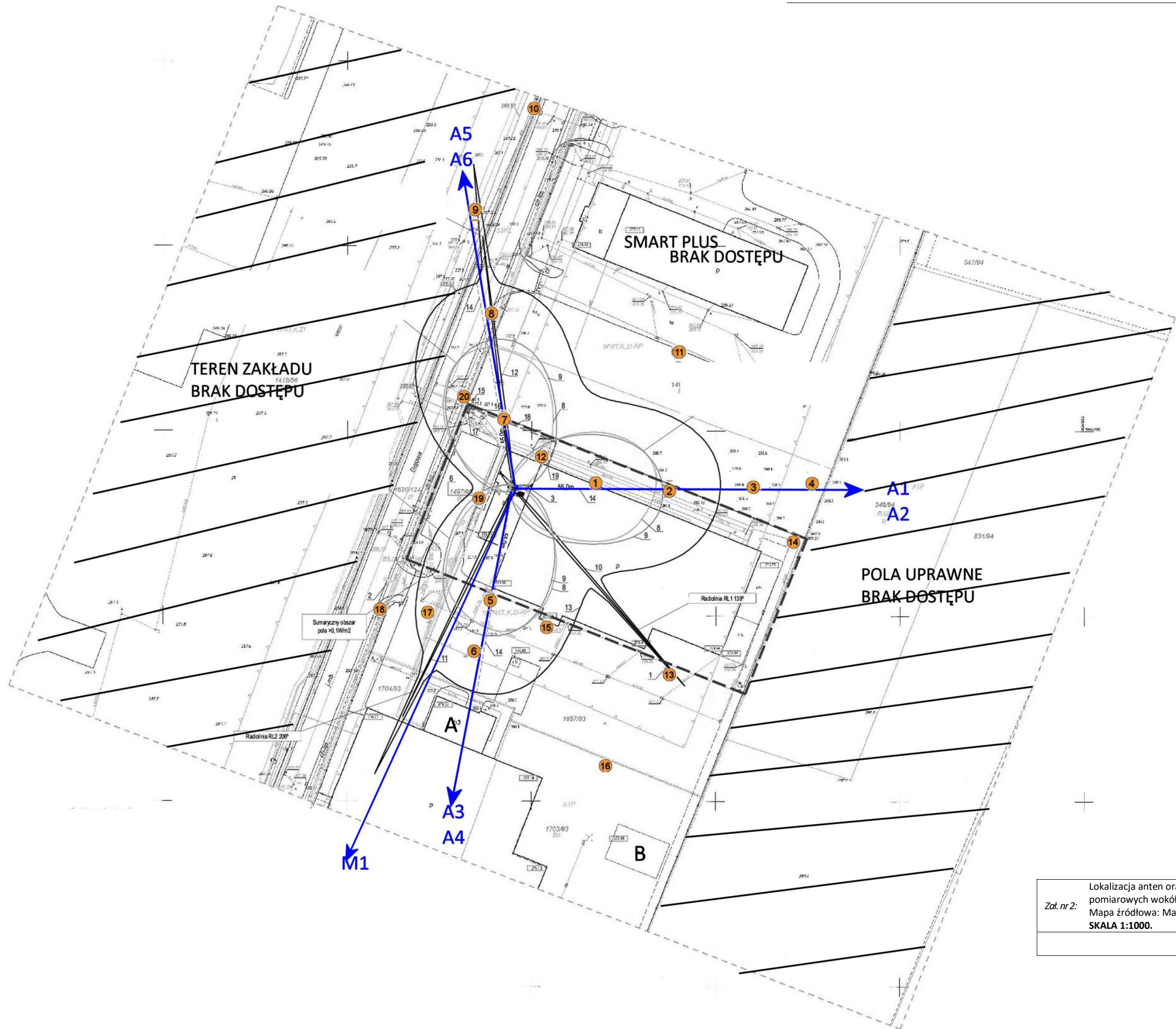
Azymuty anten
